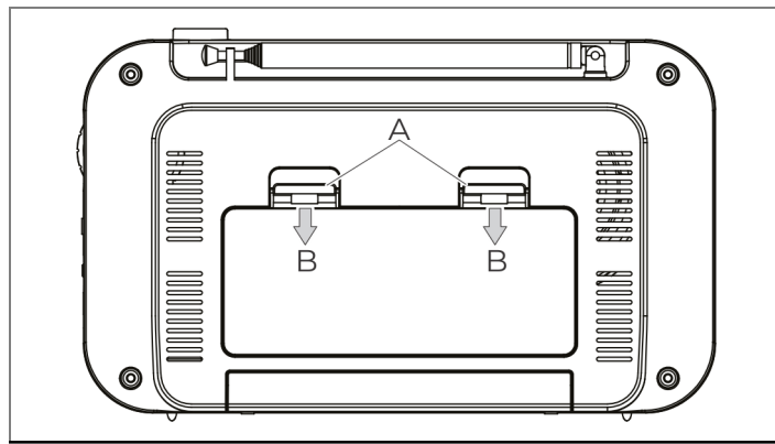
Abb. 3: Batteriefach öffnen
